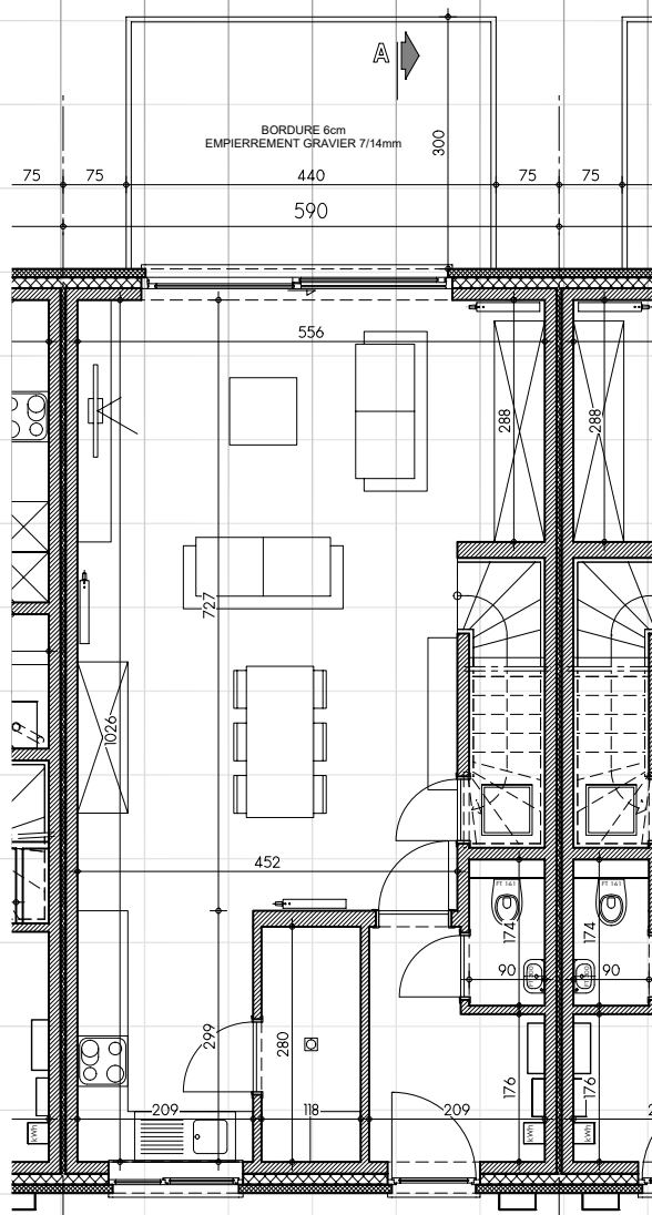
Rez-de-chaussée
